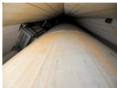
△東京スカイツリー内部の構造物 「心柱」
